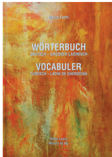
Fig. 4: Wörterbuch Deutsch–Grödner-Ladinisch
